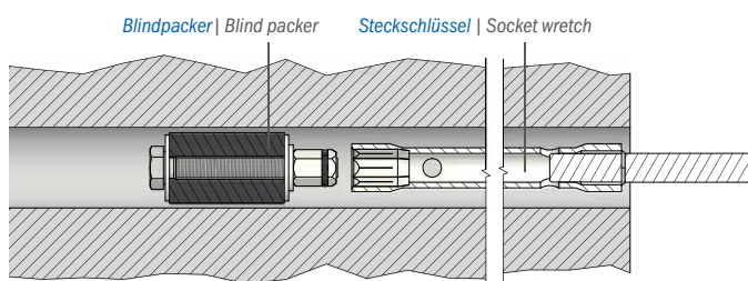
TW-Blindpacker spannen auch in großen Tiefen mit Akkuschauber TW blind packers clamp even at great depths with cordless screwdriver
